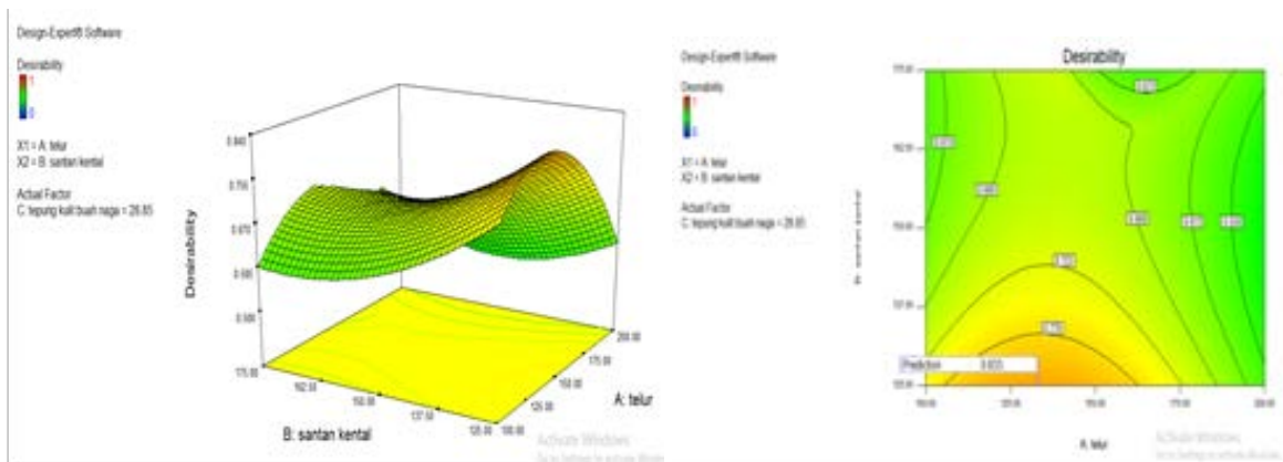
Gambar 5. Grafik Permukaan Respon, Kontur, dan Titik Optimum Variabel Kualitas Respon
